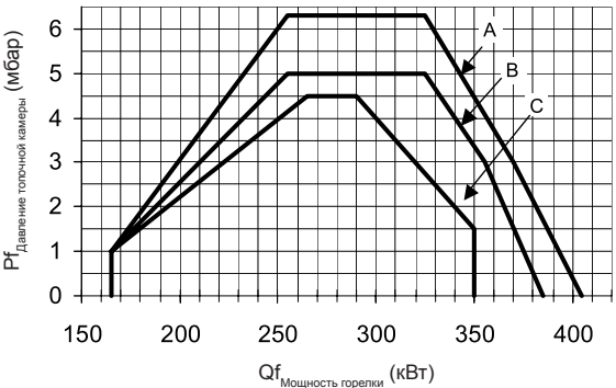
A : EG 03B.400 R2G G20 300 мбар B : EG 03B.400 R2G G20 20 мбар C : EG 03B.400 F2G 37 мбар
